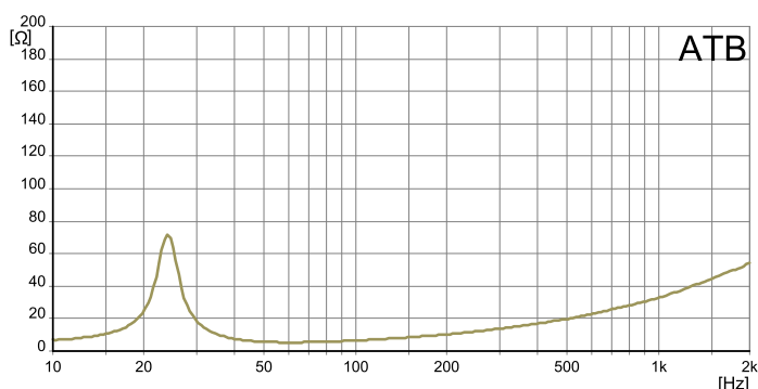
Impedanzverlauf / Impedance
