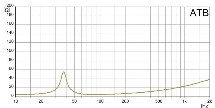
Impedanzverlauf / Impedance
